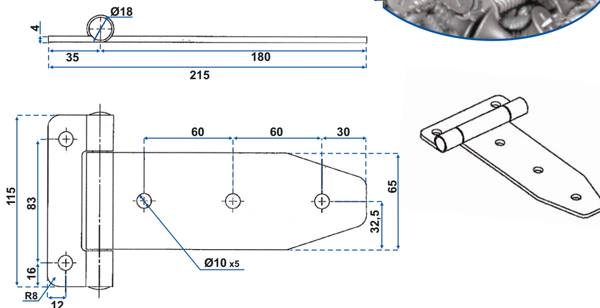
Cerniera laterale INOX AISI-316L mm.215x115
